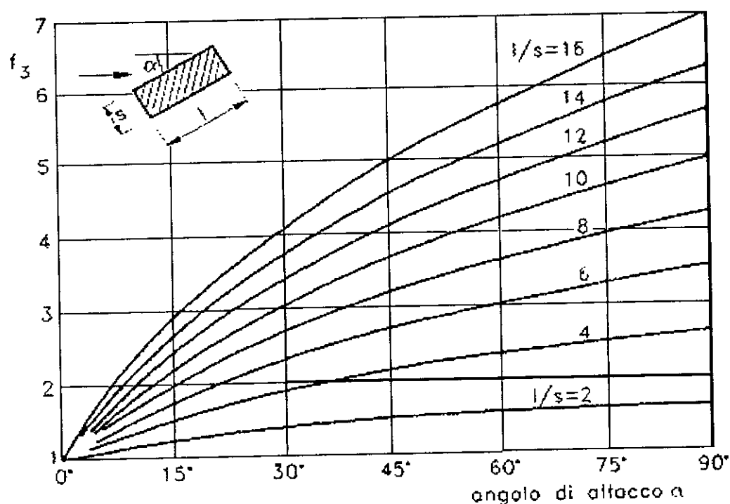
Fig. 4: funzione f_3(\alpha, l/s)
